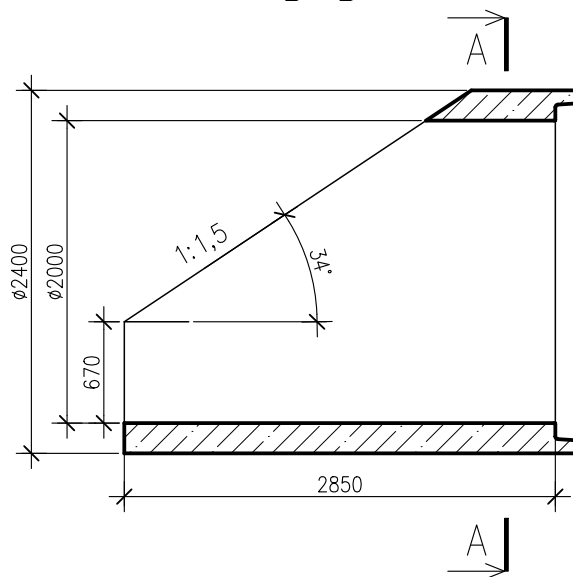
PRZEKRÓJ B-B
